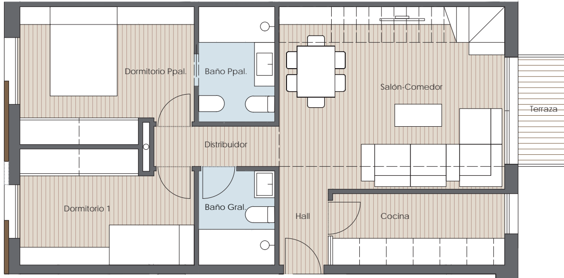
VIVIENDA DÚPLEX TIPO 03 PLANTA INFERIOR
