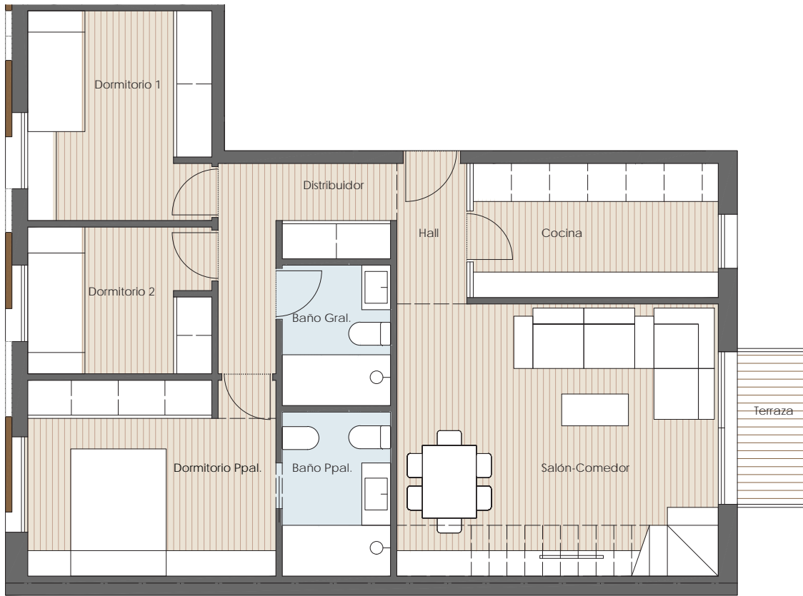
VIVIENDA DÚPLEX TIPO 04 PLANTA INFERIOR
