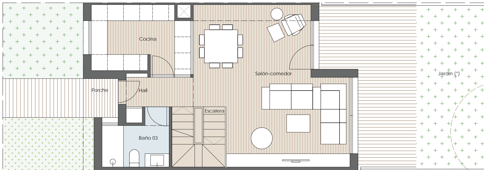
PLANTA BAJA
